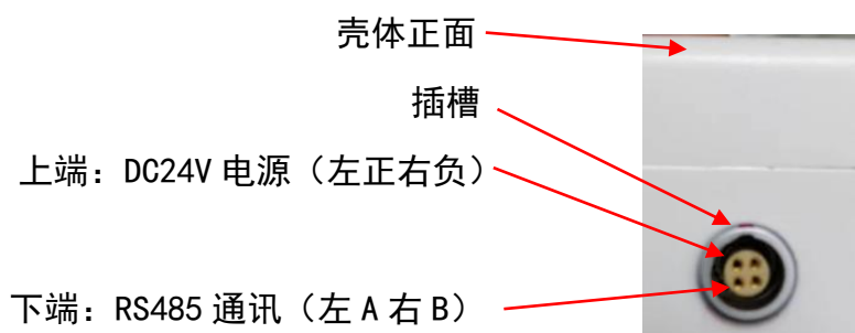
图 12. 智能温振传感器有线通讯的插接口
