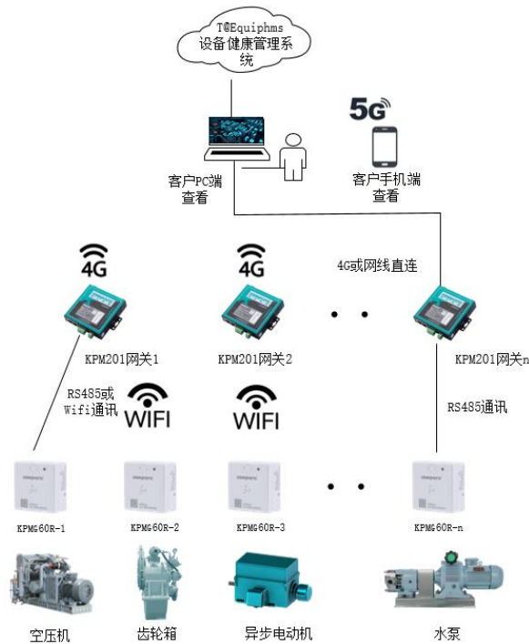
图 1. 系统拓扑图
