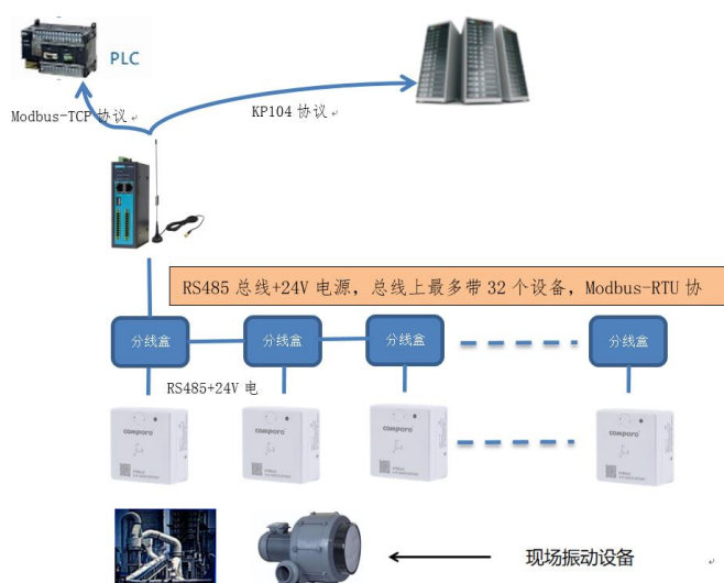
图 13. 智能温振传感器有线通讯的接线方案
