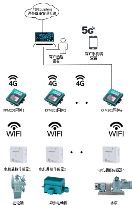
图 1. 系统拓扑图
